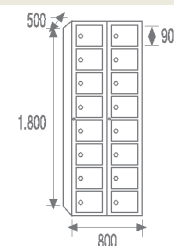
STV8-40/2 COD. 44082
