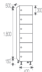
FB-40/C COD. 53062
