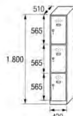
LM-40/1 COD. 74031
