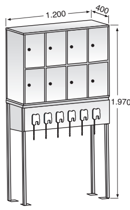
4 CSVS2P + 1 MA1200
