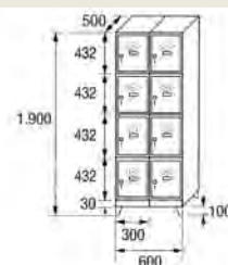
SC-30/2 COD. 43022
