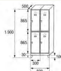
ST-30/2 COD. 43012
