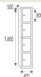
STV4-40/1 COD. 44041
